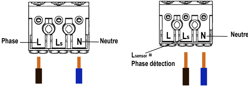
Schéma de câblage hublot en ON/OFF
