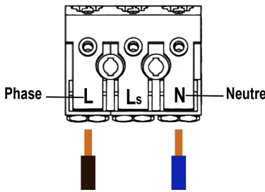
Schéma de câblage hublot en ON/OFF
