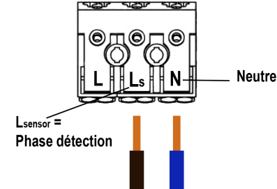
Schéma de câblage hublot avec détection
