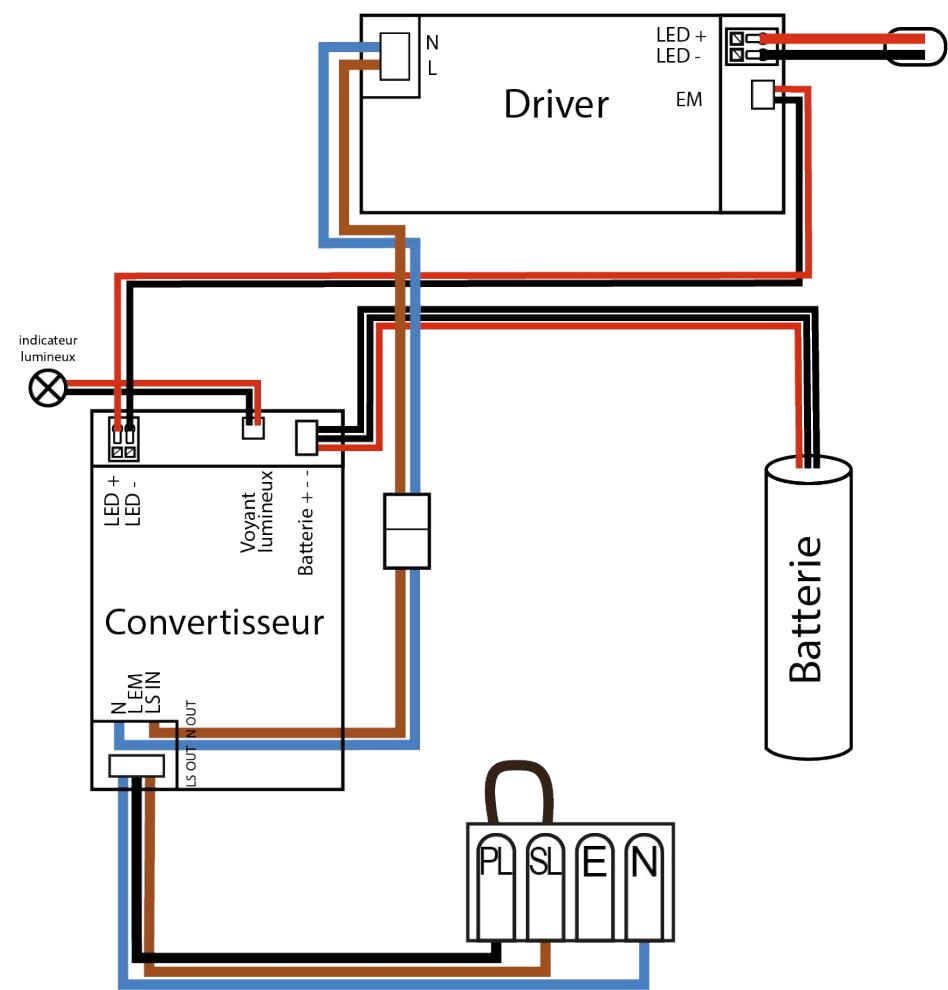
Schéma de câblage option kit de secours:
