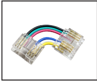
188051 Connecteur angle pour ruban 24V COB RGBWW
