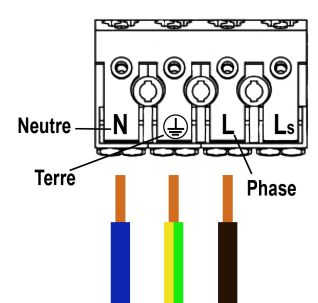
Schéma de câblage hublot en ON/OFF
