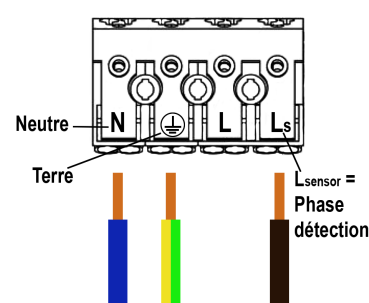
Schéma de câblage hublot avec détection
