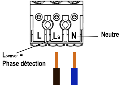
Schéma de câblage hublot avec détection
