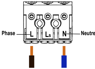
Schéma de câblage hublot en ON/OFF
