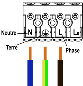
Schéma de câblage hublot en ON/OFF
