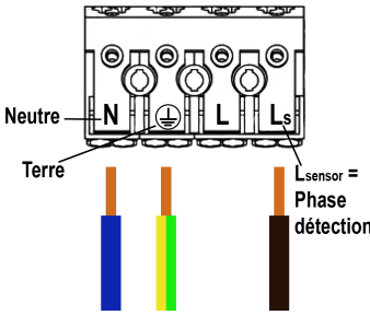
Schéma de câblage hublot avec détection
