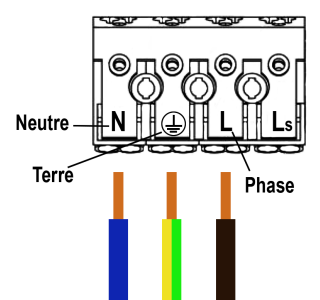
Schéma de câblage hublot en ON/OFF
