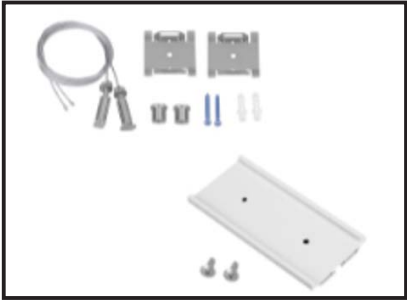
Patte saillie / kit de suspension / plaque de jonction
