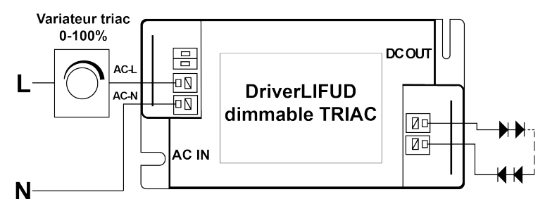
Schéma de câblage de la gradation TRIAC
