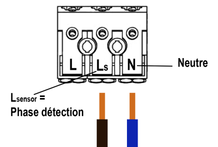
Schéma de câblage hublot avec détection
